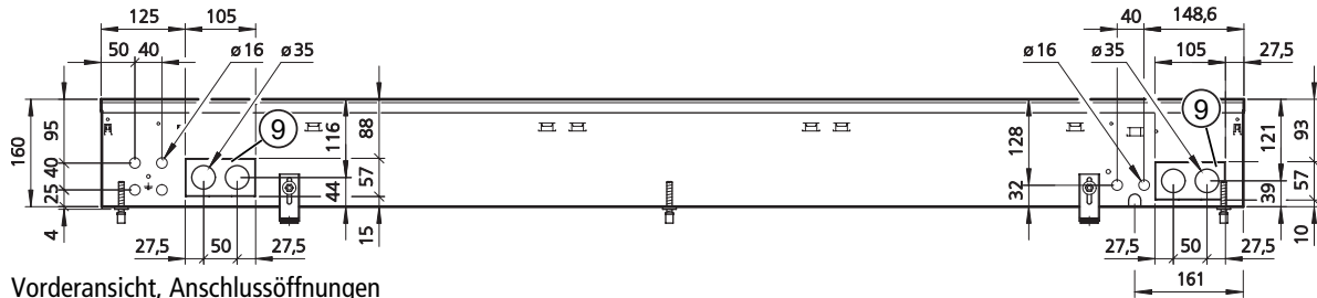
Vorderansicht, Anschlussöffnungen
