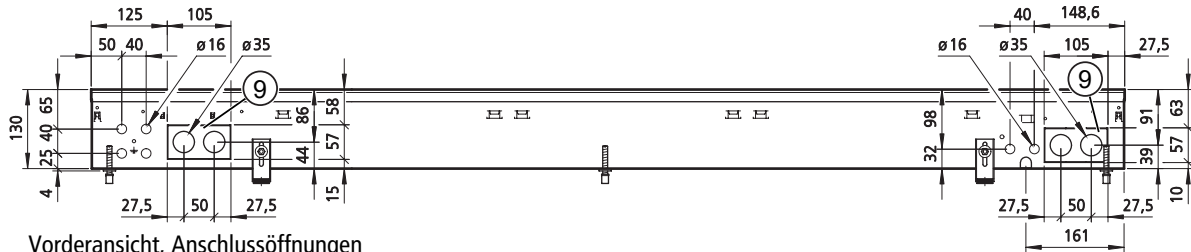
Vorderansicht, Anschlussöffnungen
