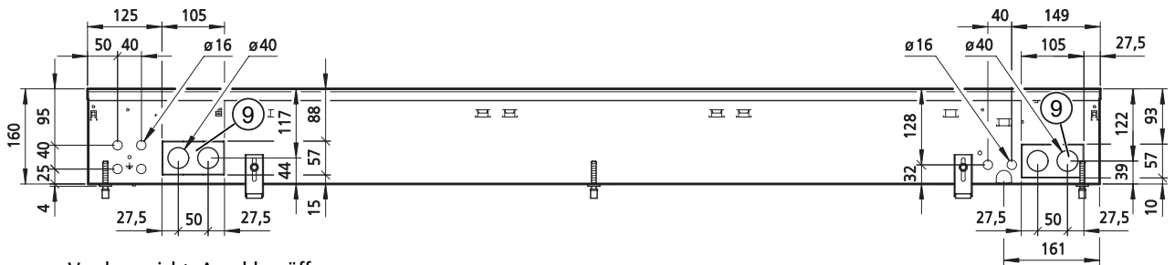
Vorderansicht, Anschlussöffnungen
