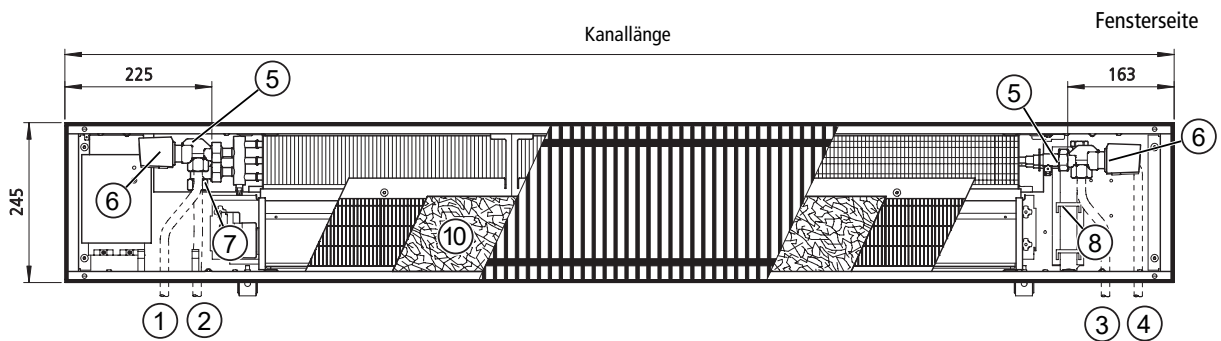
Draufsicht, Wasseranschluss raumseitig
