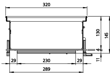
Abb. 8: Bsp.: HK 320, HK 320 E, H = 130 mm, 2-Leiter, vergrößerte Kanalhöhe mit Kondensatpumpe*
