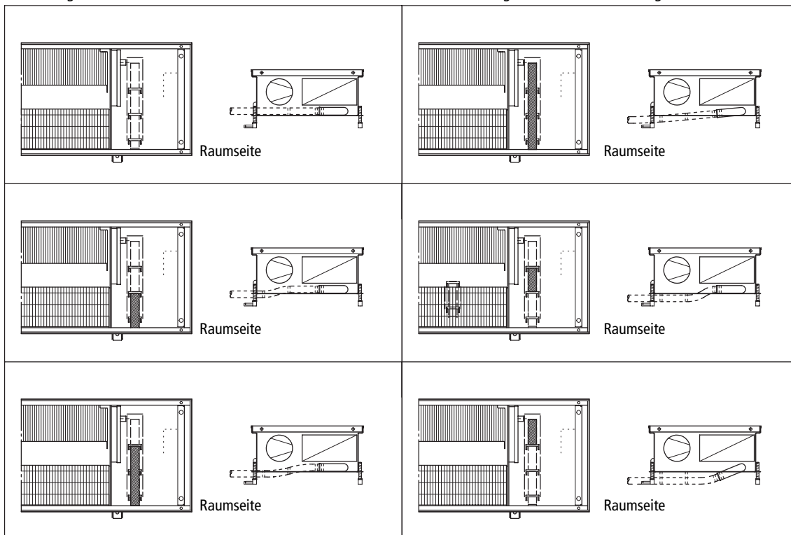
Abb. 4: Möglichkeiten zur Herausnahme der Bodenblech-Ausschnitte und Verlegung der bauseitigen Kondensatableitung
