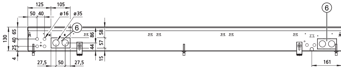
Vorderansicht, Anschlussöffnungen
