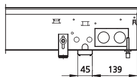
Vorderansicht mit eingebauter Kondensatpumpe
