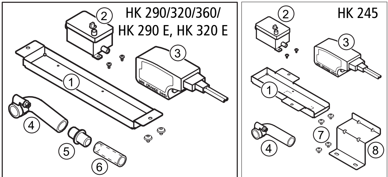
Abb. 6: Anbausets
