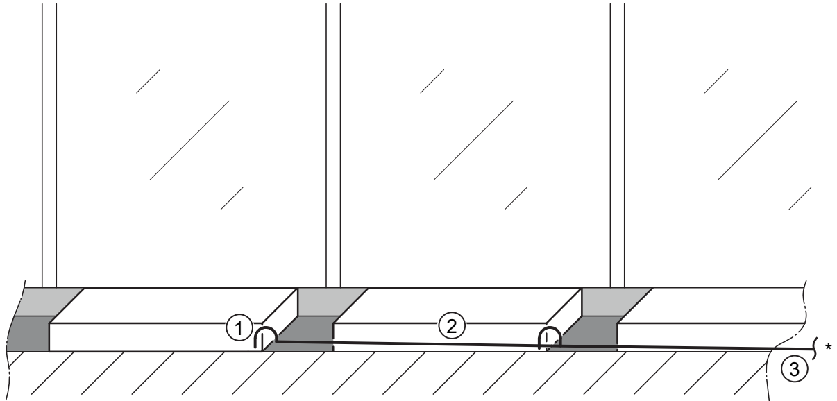
Bauseitige Kondensatabführung mit Kondensatpumpe
