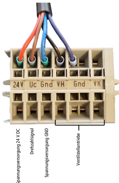
Abb. 9: Anschluss elektromechanisch (*24), Katherm HK 320/130, 245/160, 290/160
