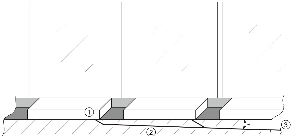
Bauseitige Kondensatabführung mit natürlichem Gefälle
