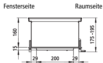
Seitenansicht mit eingebauter Kondensatpumpe
