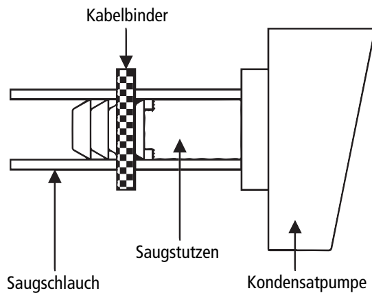
Abb. 5: Saugschlauch fixieren
