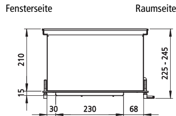
Seitenansicht mit eingebauter Kondensatpumpe
