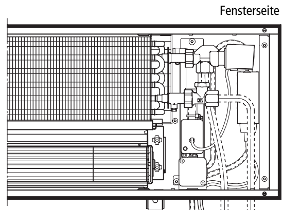
Abb. 8: Bsp.: HK 320, HK 320 E, H = 130 mm, 2-Leiter, vergrößerte Kanalhöhe mit Kondensatpumpe*
