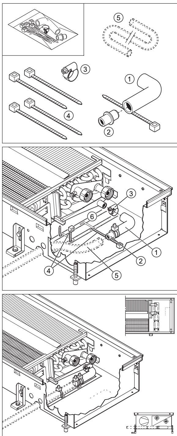
Abb. 3: Anbauset Kondensatablauf
