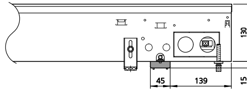
Abb. 8: Bsp.: HK 320, HK 320 E, H = 130 mm, 2-Leiter, vergrößerte Kanalhöhe mit Kondensatpumpe*
