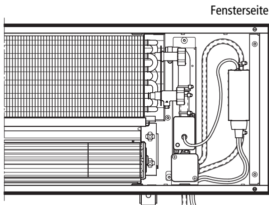
Abb. 8: Bsp.: HK 320, HK 320 E, H = 130 mm, 2-Leiter, vergrößerte Kanalhöhe mit Kondensatpumpe*
