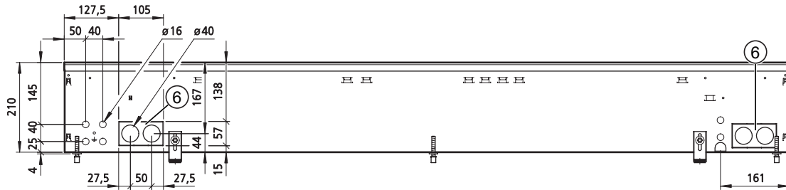
Vorderansicht, Anschlussöffnungen
