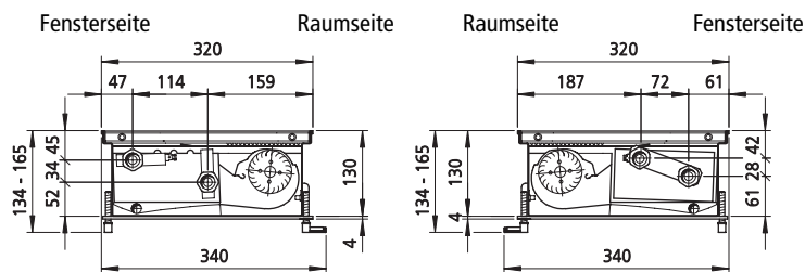
Schnitt (Kühlen oder Heizen) Beispiel: Roll-Rost
