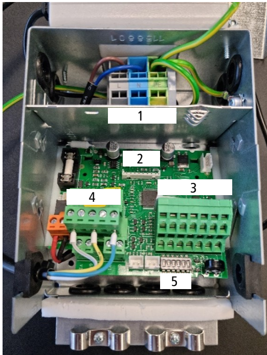
Anschlussdose für HK 320/130, 245/160, 360/210
