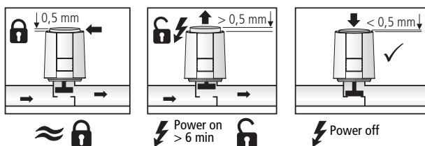
Abb. 2: "First-Open"-Funktion
