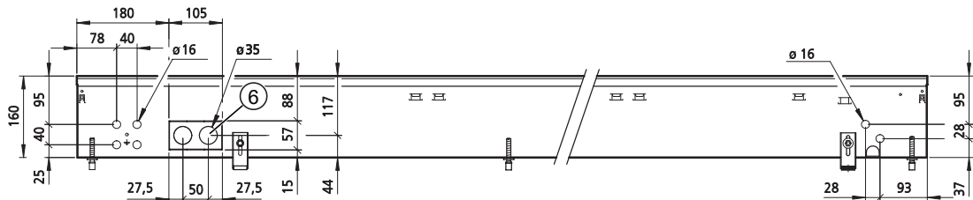
Vorderansicht, Anschlussöffnungen
