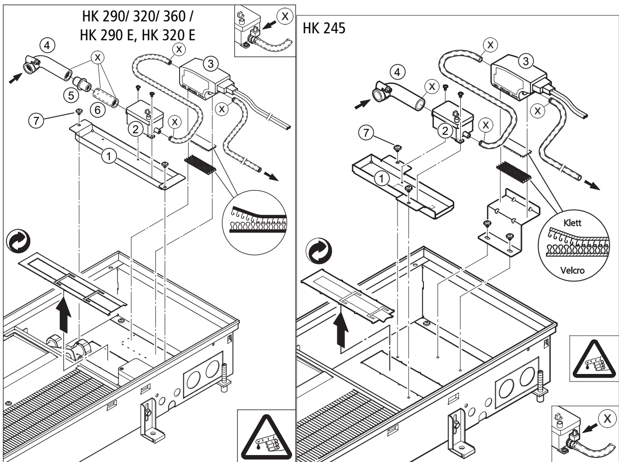
Abb. 7: Einbau Anbauset Kondensatpumpe
