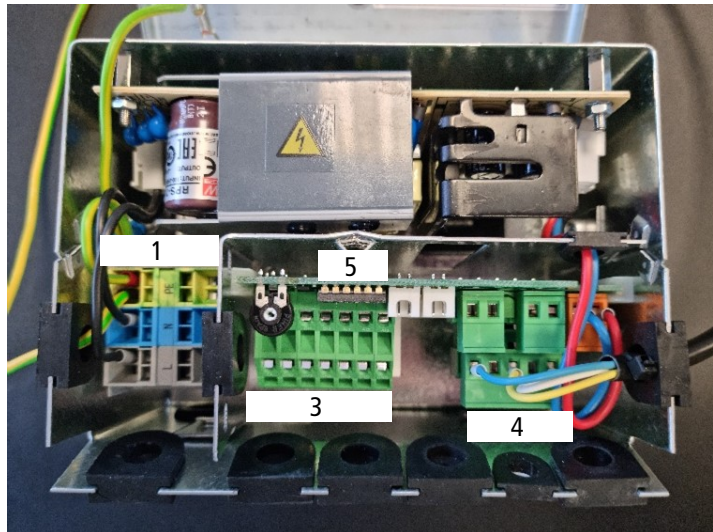
Anschlussdose für HK 290/ 160
