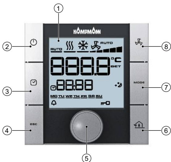
Abb. 22: KaController mit Funktionstasten, Typ 3210002
