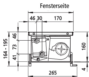
Schnitt (Kühlen oder Heizen) Beispiel: Roll-Rost
