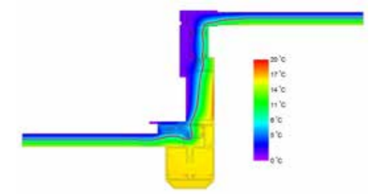
Isothermenverlauf Doppelklappe esserlux® therm: Einbaurahmen und Klappenprofile thermisch getrennt
