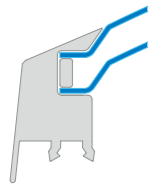
2-schalig U c -Wert 2,7 W/m 2 K U up -Wert 2,5 W/m 2 K
