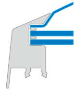
thermoplan 1 Schale, 2 Stegplatten U c -Wert 0,83 W/m 2 K U up -Wert 1,1 W/m 2 K
