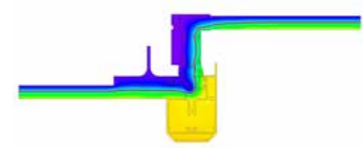
Isothermenverlauf Einzelklappe esserlux® therm: Einbaurahmen und Klappenprofile thermisch getrennt
