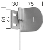
Universalträger mit Seilführung
