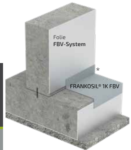
mit Bodenplattenüberstand
