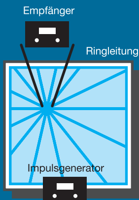
Bild: Nass-Ortungsverfahren
