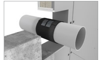
Fertige Wicklung mit Gewebiband und an den Außenseiten mit Kabelbindern fixieren s.u.
