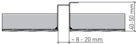
Kassettenlängsfuge mit Distanzierung (Typ A/C) Tile longitudinal joint with spacer (Type A/C)
