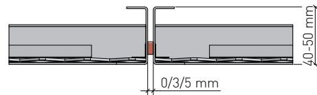
Kassettenlängsfuge mit Dichtband bei Kassetten aus Blech mit Streckgitter eingelegt und fixiert (Typ C) Tile longitudinal joint with embossing on sheet metal tiles with expanded metal mesh inserted and fixed (Type C)
