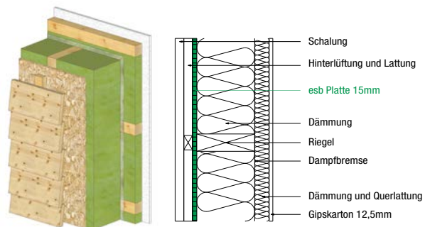
Außenwand 2 – hinterlüftet
